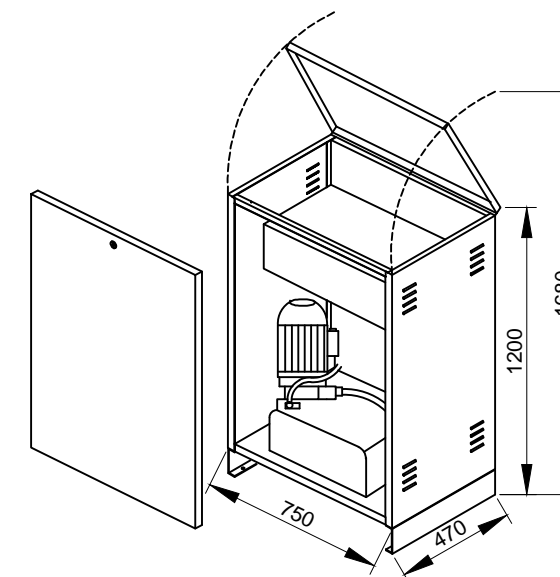
Machinekamer SCHAAL 1:30
